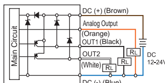
AP50 □ - 031 - □ 2 PNP + Analog Output(4~20mA)
