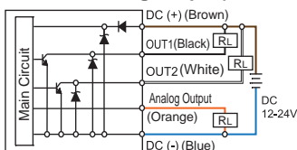
AP50 □ - 011 - □ 2 NPN + Analog Output(4~20mA)
